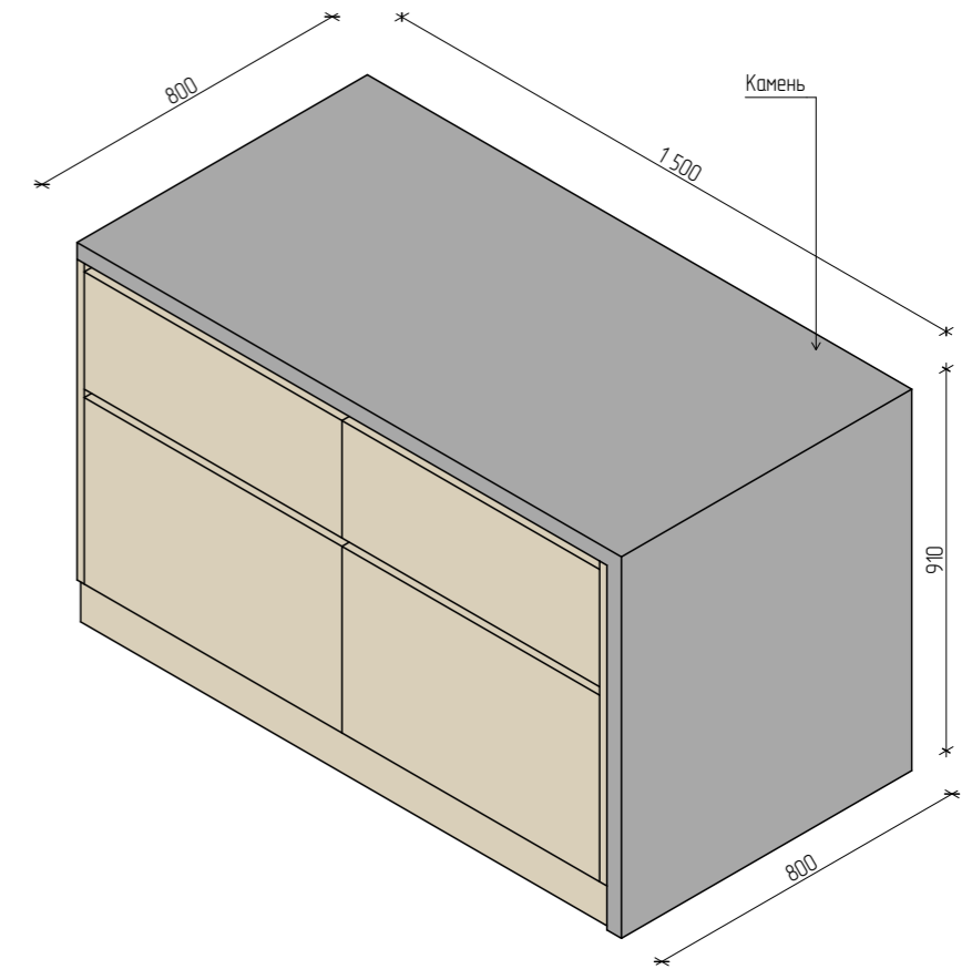
Аксонометрия. Вид 2
