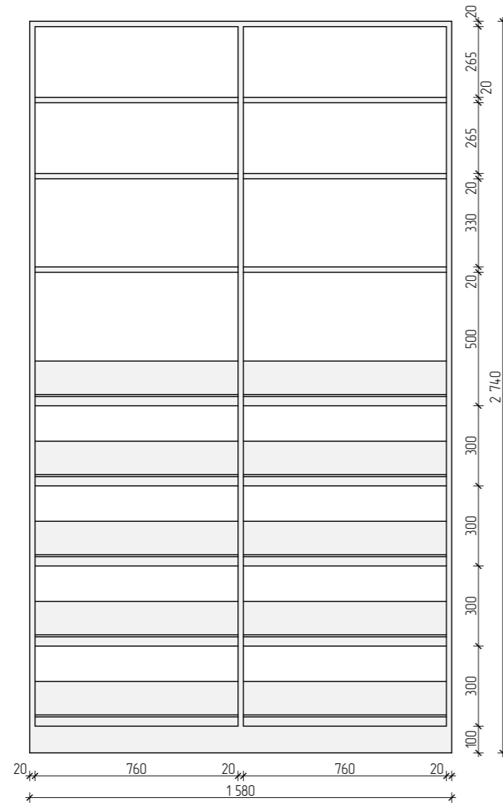
Вид спереди
