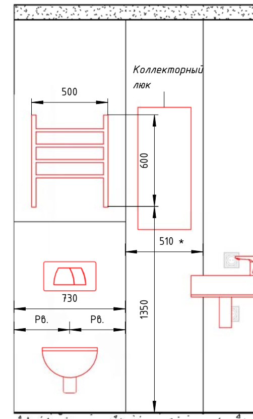
3-3 ( 1 : 25)
