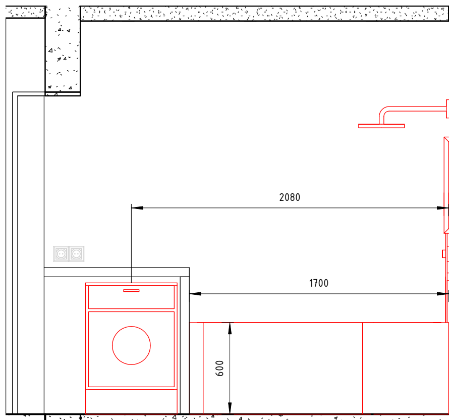
1-1 ( 1 : 25 )
