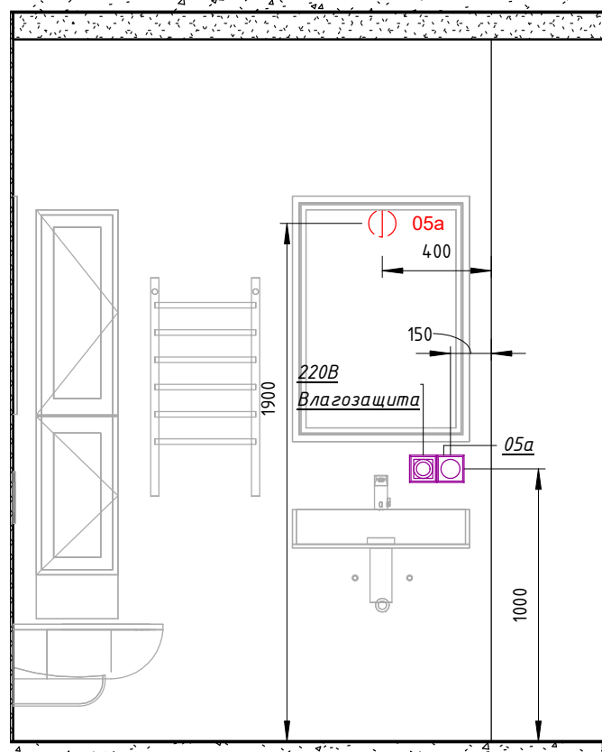
05.1 ( 1 : 25 )
