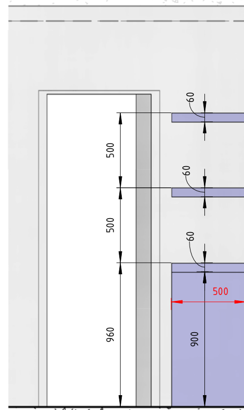
3-3 ( 1 : 25 )
