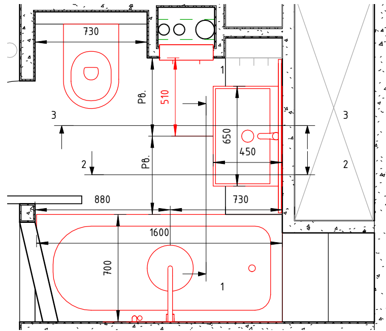
M02 План ( 1 : 25)
