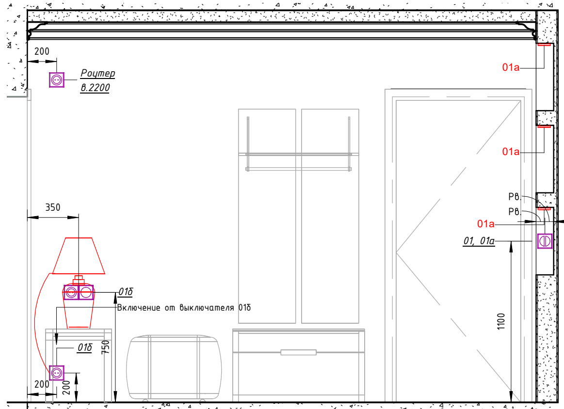
01.1 ( 1 : 25)
