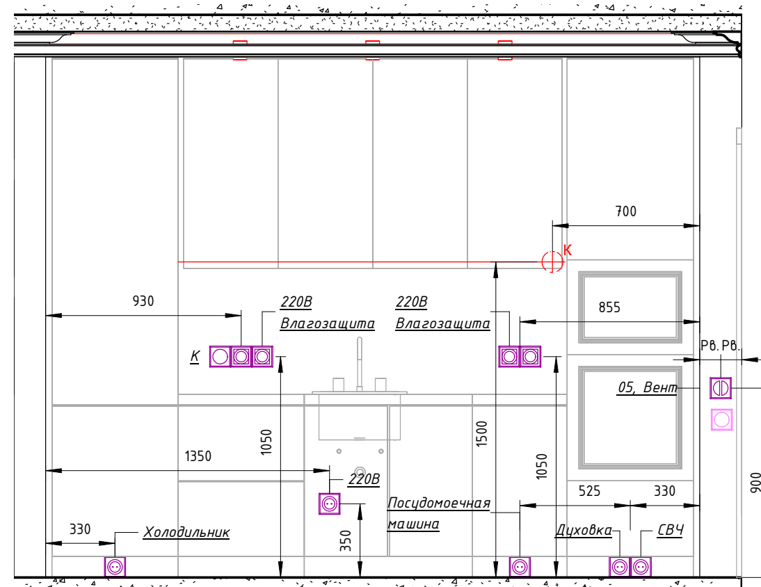
03.1 ( 1 : 25)
