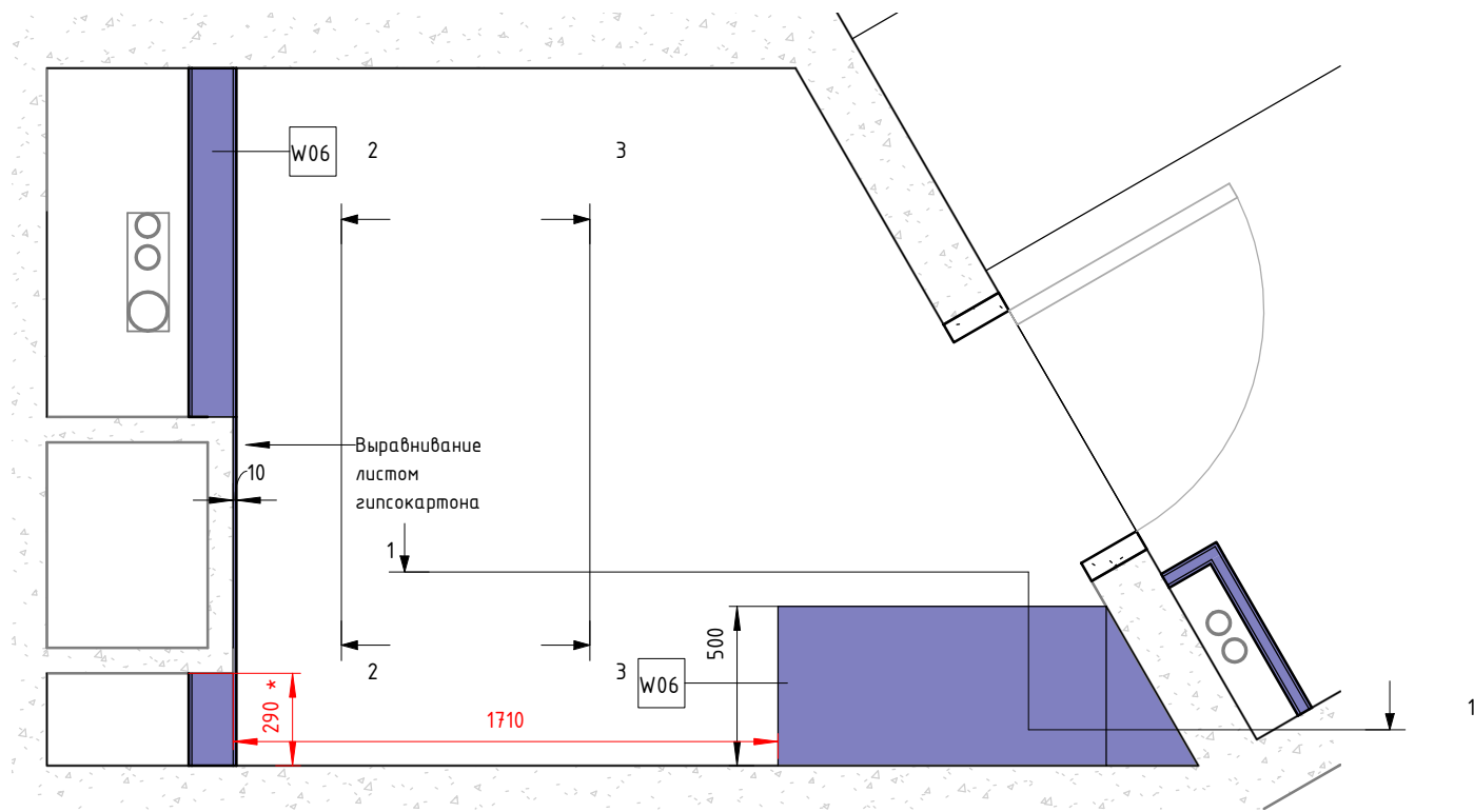
П2 ( 1 : 25 )
