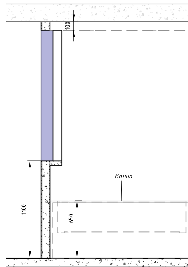
2-2 ( 1 : 25 )
