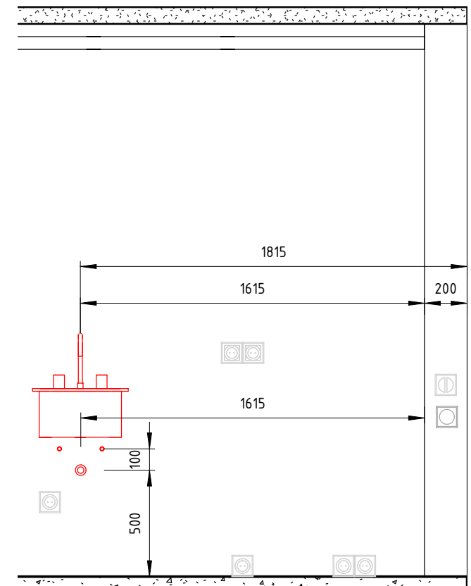
4-4 ( 1 : 25 )
