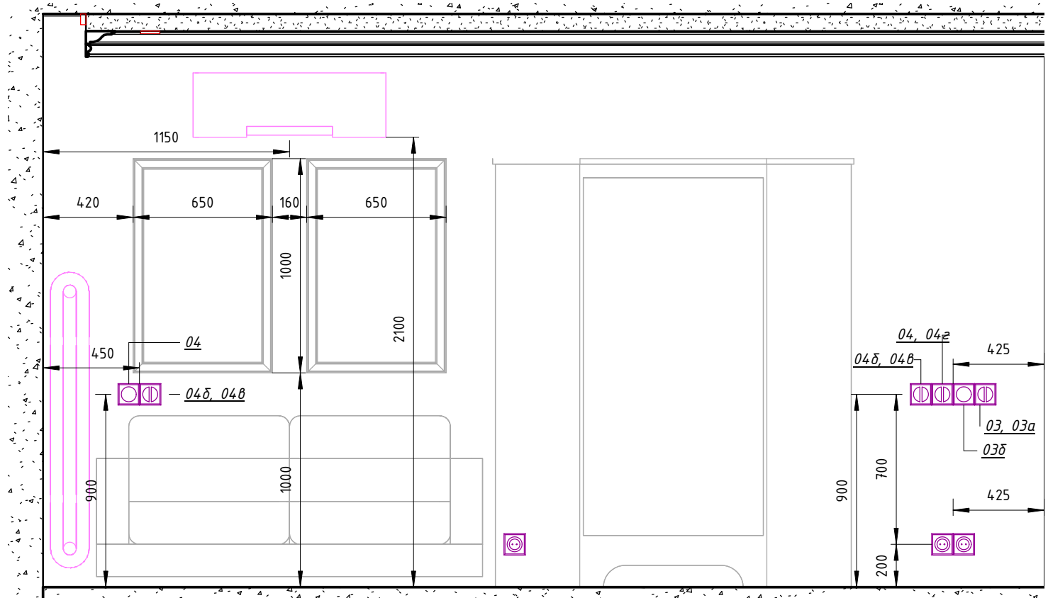
04.2 ( 1 : 25 )
