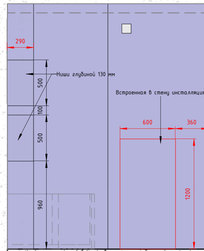
2-2 ( 1 : 25 )
