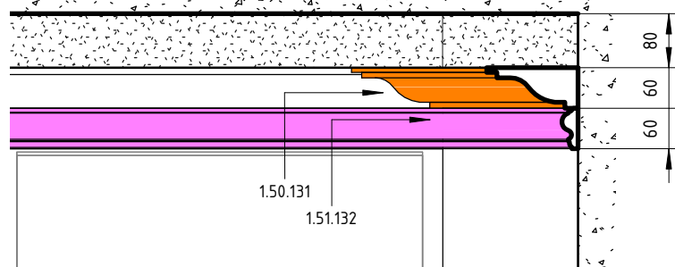
2-2 ( 1 : 10 )
