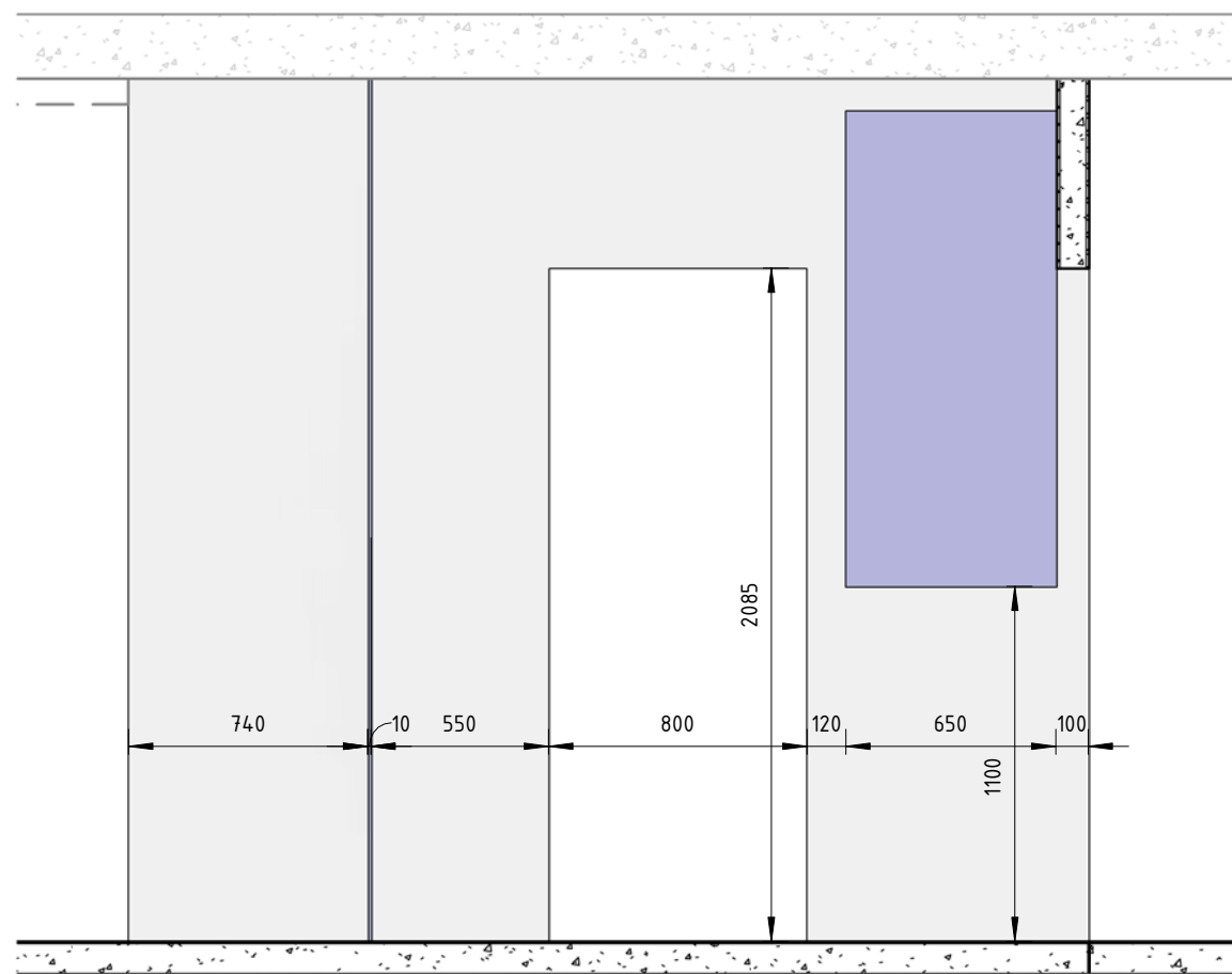
1-1 ( 1 : 25 )
