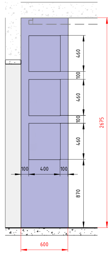
4-4 ( 1 : 25 )
