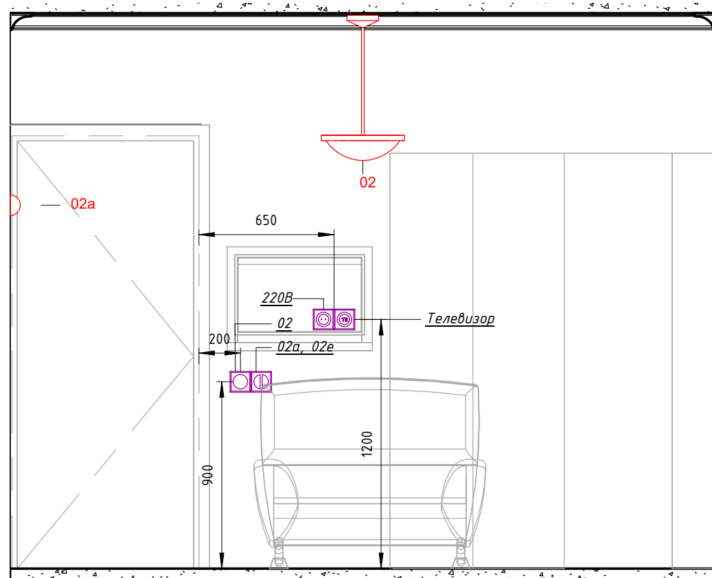
02.1 ( 1 : 25 )
