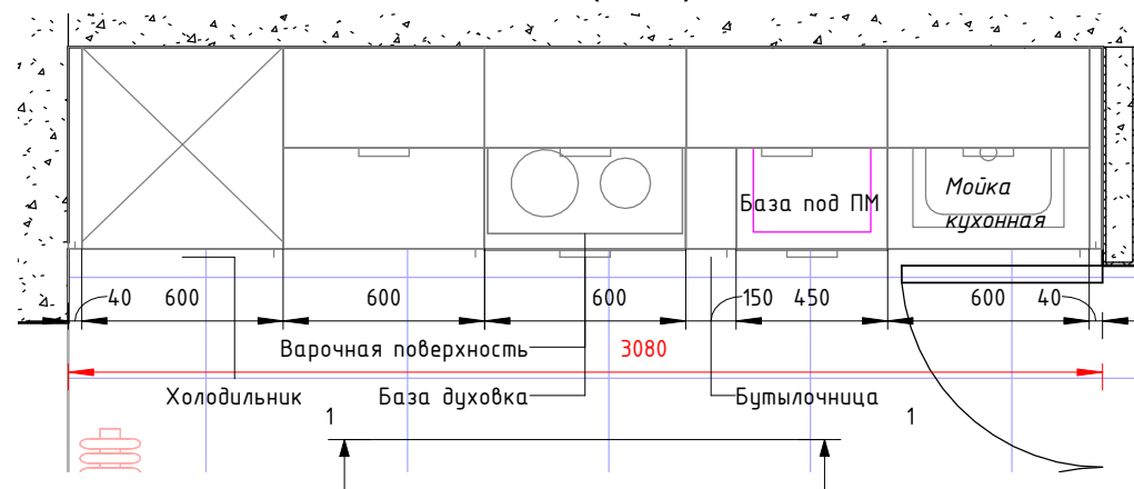
К1 План ( 1 : 25)
