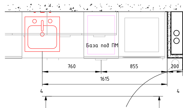
M03.2 План
