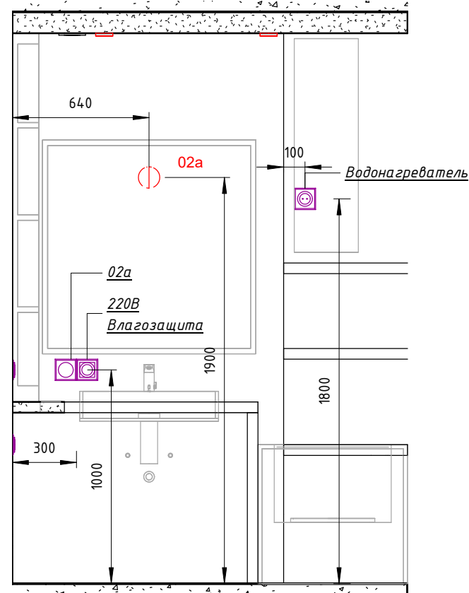
02.1 ( 1 : 25 )
