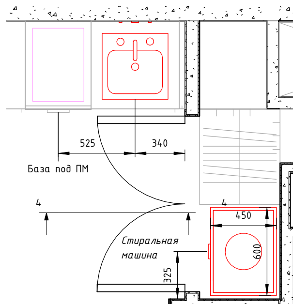
M03.1 План ( 1 : 25)
