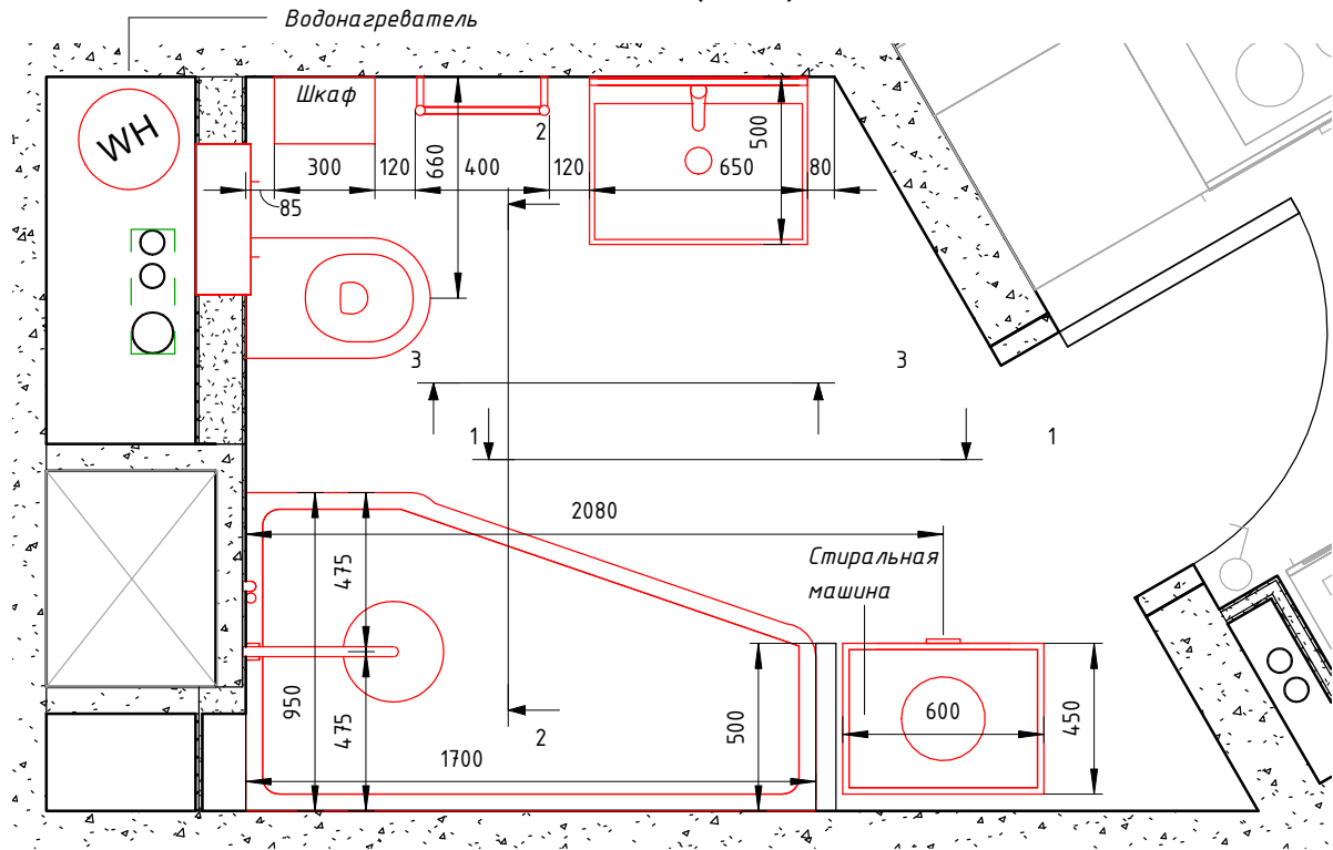
M05 План ( 1 : 25 )
