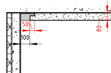
3-3 ( 1 : 25 )
