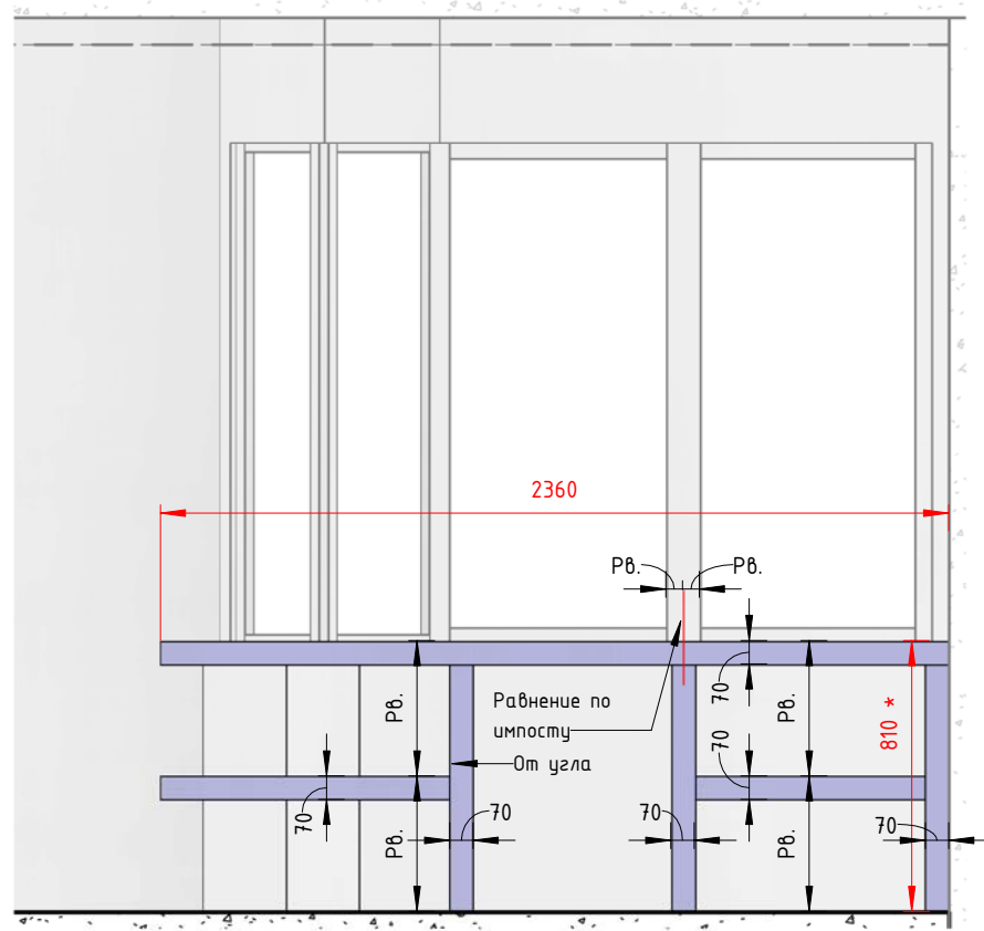
6-6 ( 1 : 25 )
