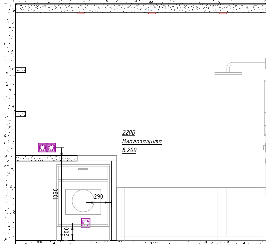
05.2 ( 1 : 25 )
