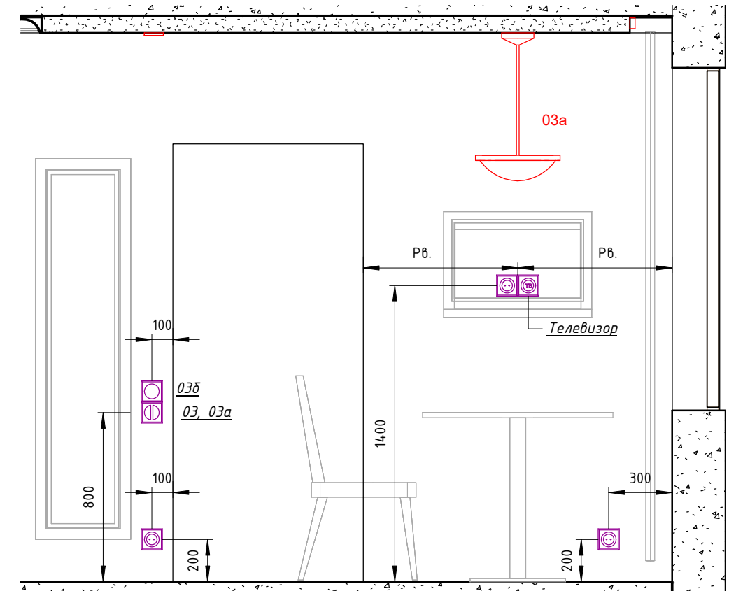
03.2 ( 1 : 25 )
