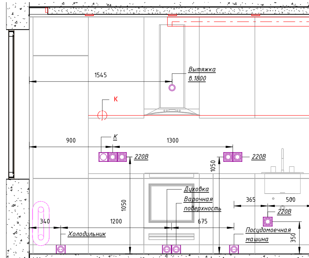
03.1 ( 1 : 25 )
