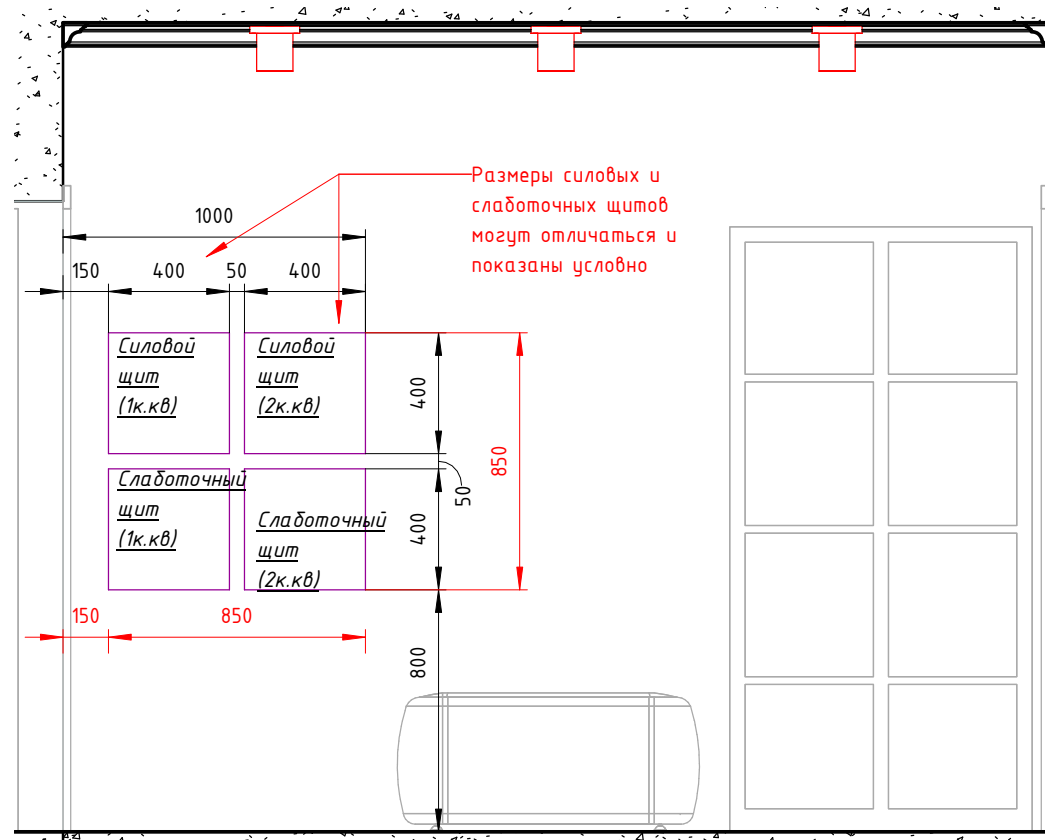
00.1 ( 1 : 25 )
