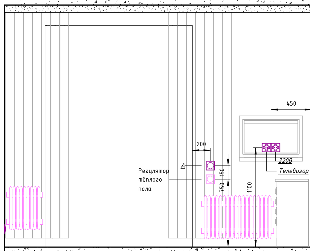
02.3 ( 1 : 25 )
