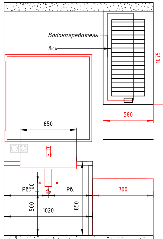
1-1 ( 1 : 25)
