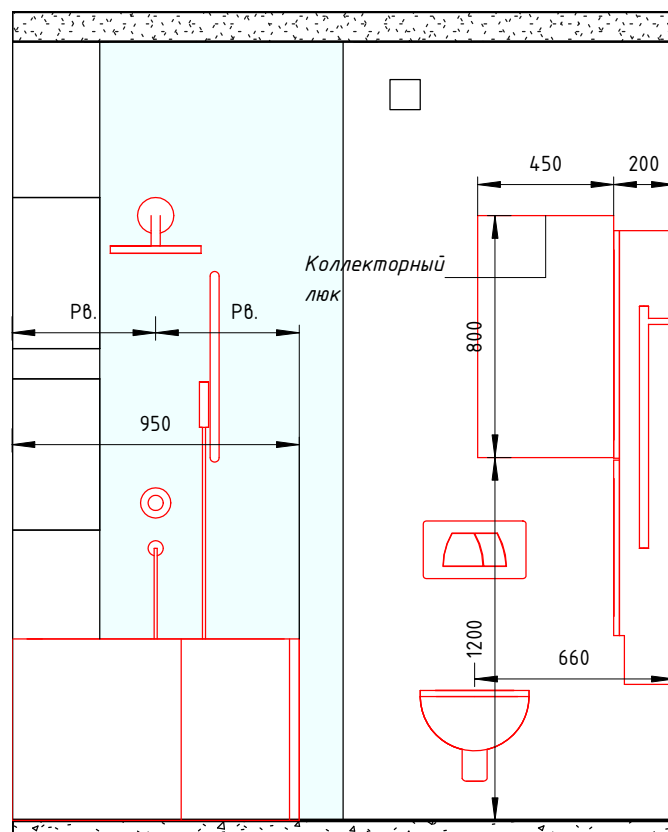
2-2 ( 1 : 25 )
