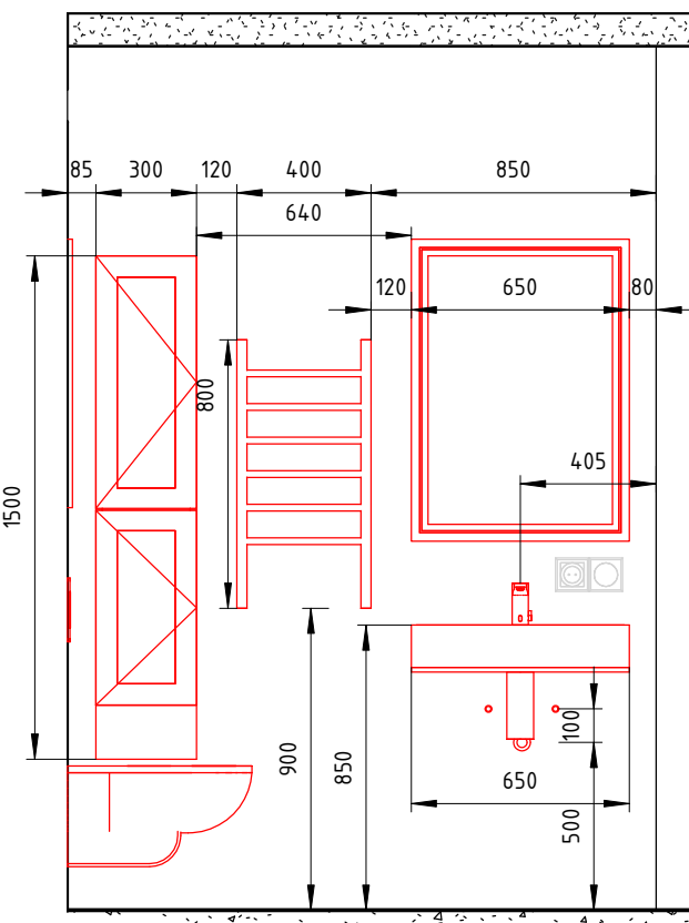
3-3 ( 1 : 25 )
