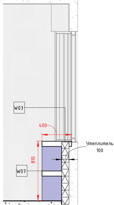
7-7 ( 1 : 25 )
