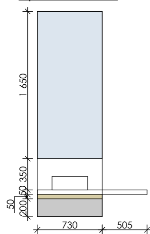
Тумба в с/у гостевой. Фронтальный вид
