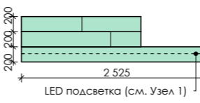
Фрагмент 6. Фронтальный вид
