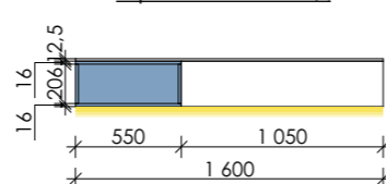
Тумба в с/у для мальчика. Фронтальный вид
