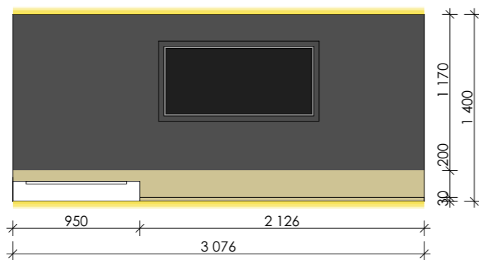
Зона ТВ. Фронтальный вид
