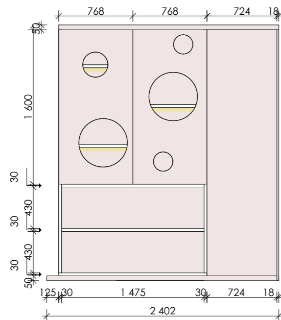
Стеллаж. Фронтальный вид. Фасады
