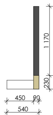
Зона ТВ. Вид сбоку
