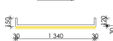
Полка над кроватью. Вид сбоку
