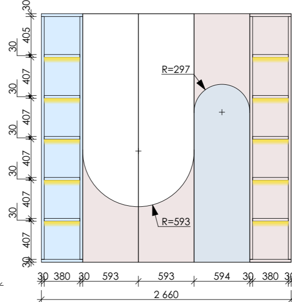
Шкаф. Фронтальный вид
