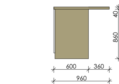
Остров. Вид сбоку
