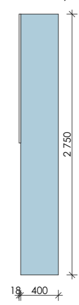
Пенал в с/у для девочки. Вид сбоку
