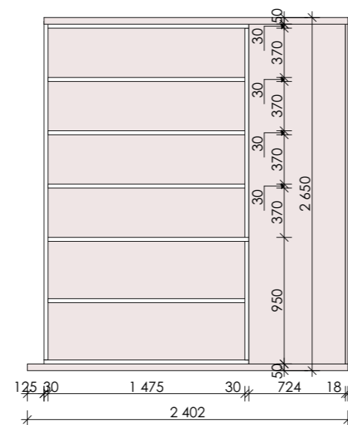
Стеллаж. Фронтальный вид. Внутри
