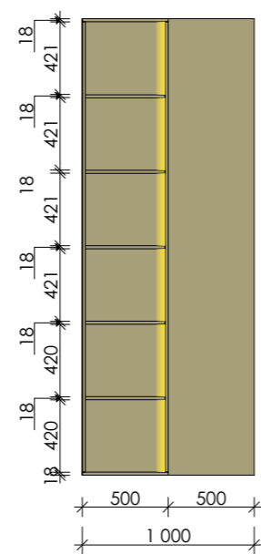
Стеллаж. Фронтальный вид
