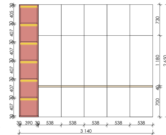
Шкаф. Фронтальный вид
