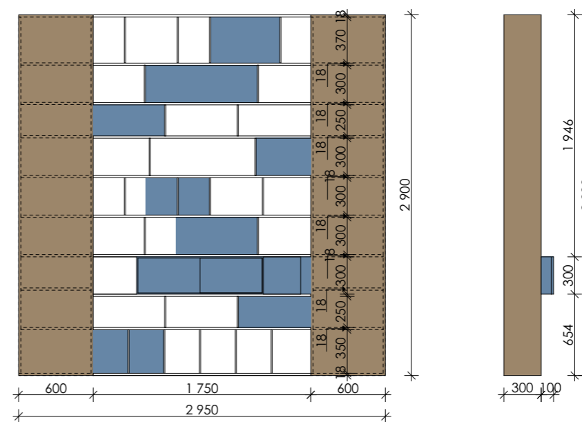
Стеллаж. Фронтальный вид
