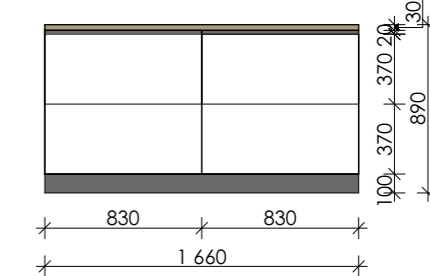
Остров. Фронтальный вид
