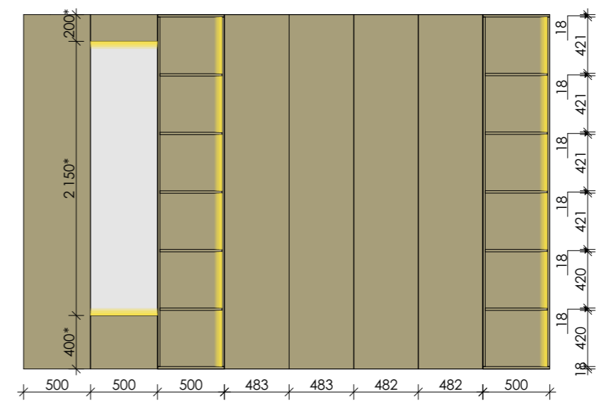
Стеллаж. Фронтальный вид
