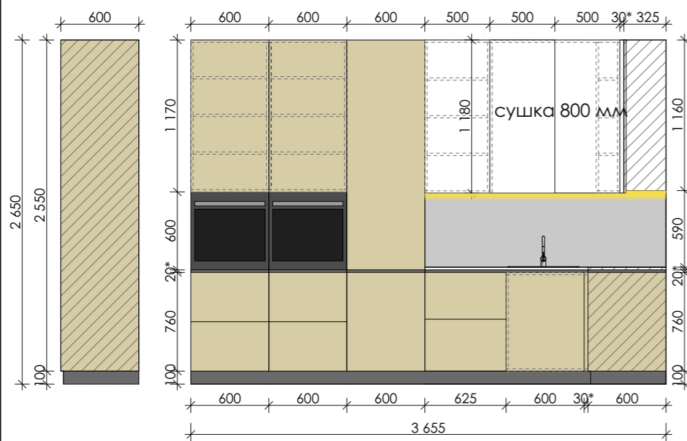
Кухня. Вид сбоку 1
