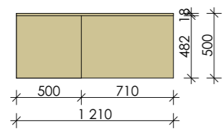
Тумба Фронтальный вид
