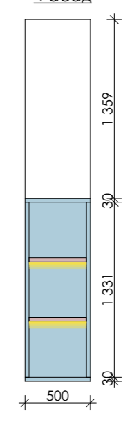
Пенал в с/у для девочки. Фронтальный вид.
